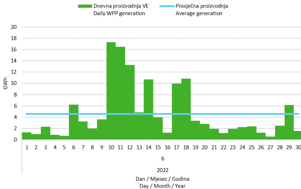
Slika 5 Dnevna proizvodnja svih vjetroelektrana u lipnju 2022. godine Figure 5 Daily generation of all wind power plants in June 2022
