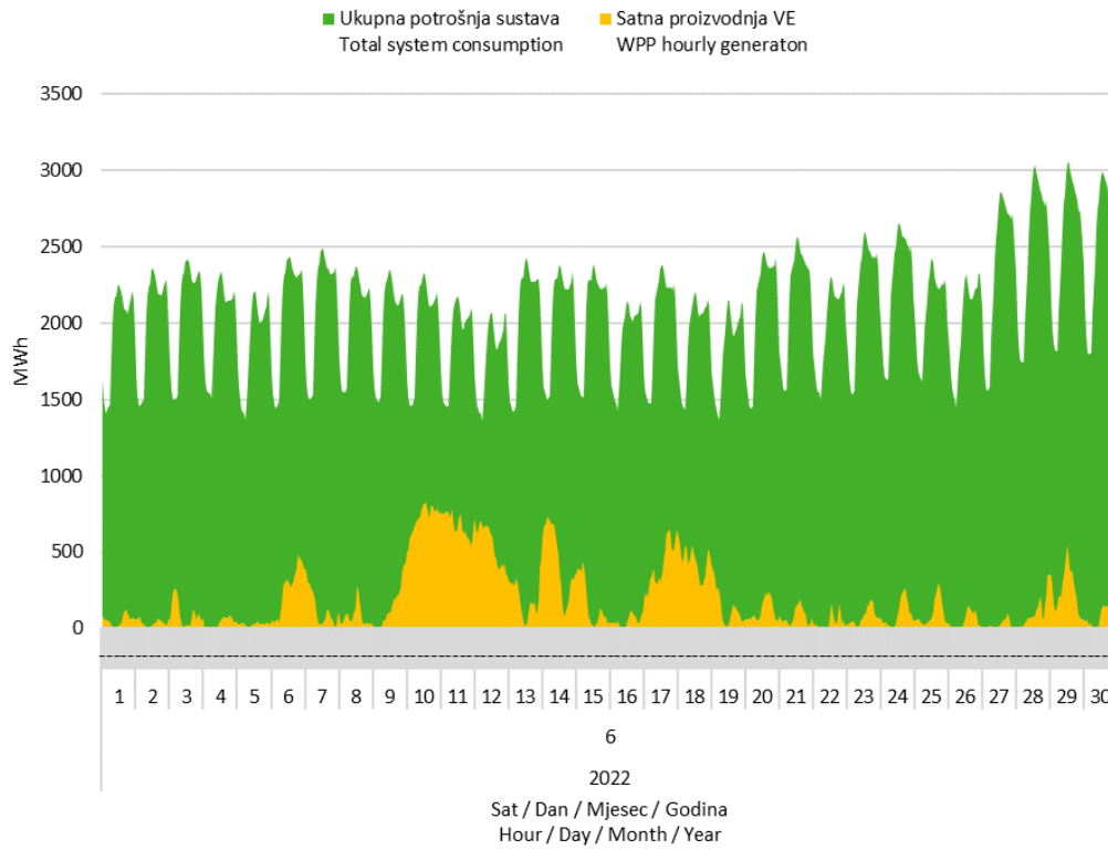
Slika 7 Usporedba satnog dijagrama opterećenja sustava i proizvodnje vjetroelektrana u lipnju 2022. godine
