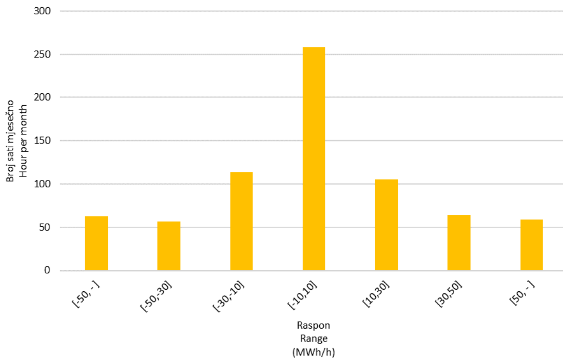
Slika 10 Statistička raspodjela satnih promjena proizvodnje VE u lipnju 2022. godine
