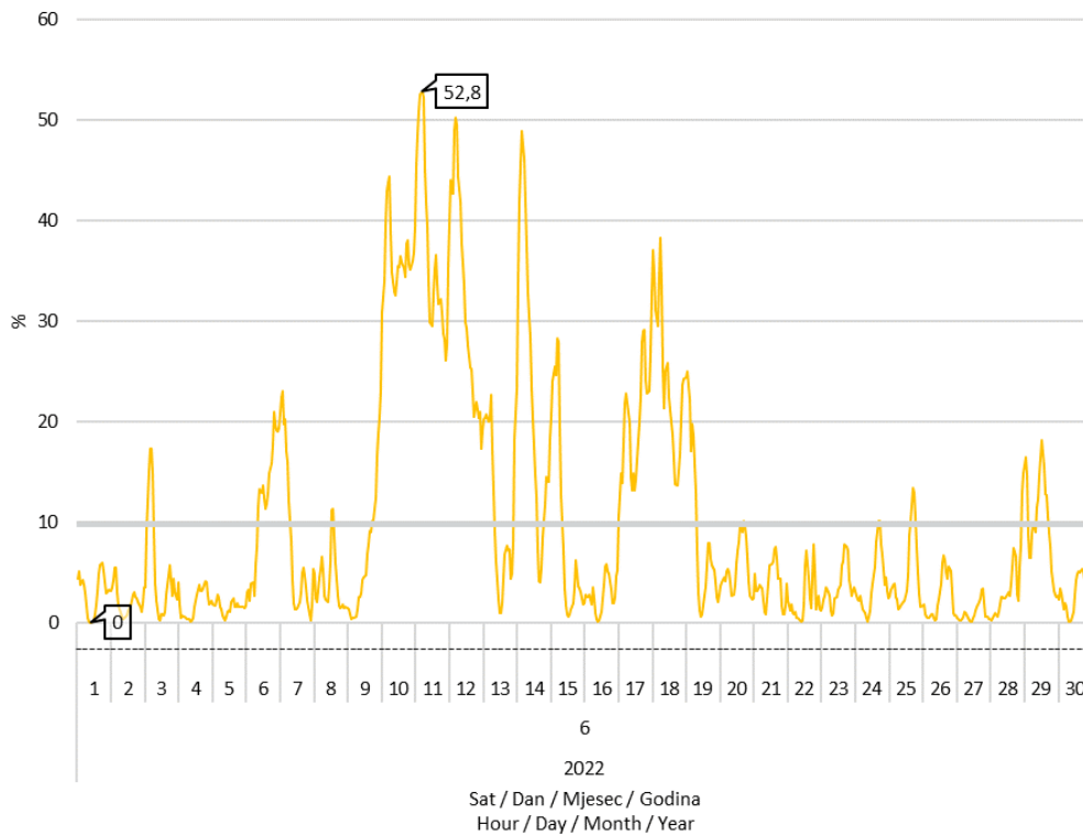
Slika 8 Udio proizvodnje vjetroelektrana u pokrivanju satnog opterećenja elektroenergetskog sustava u lipnju 2022. godine
