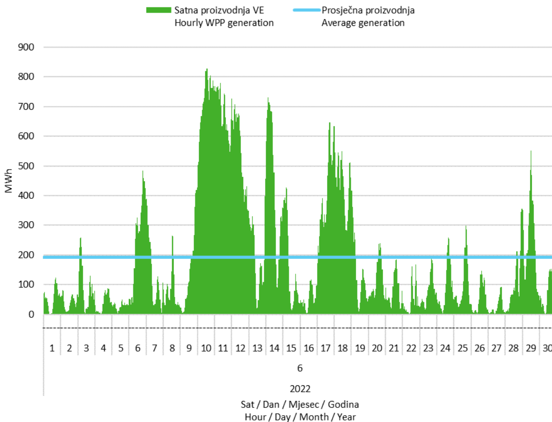
Slika 2 Satna proizvodnja svih vjetroelektrana u lipnju 2022. godine
