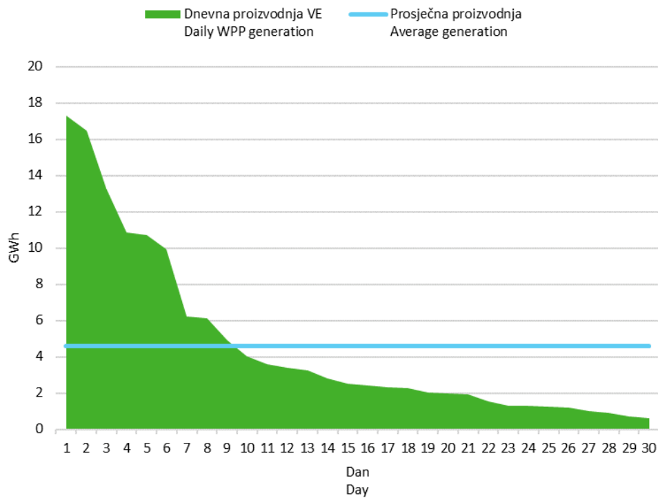
Slika 6 Krivulja trajanja dnevne proizvodnje vjetroelektrana u lipnju 2022. godine
