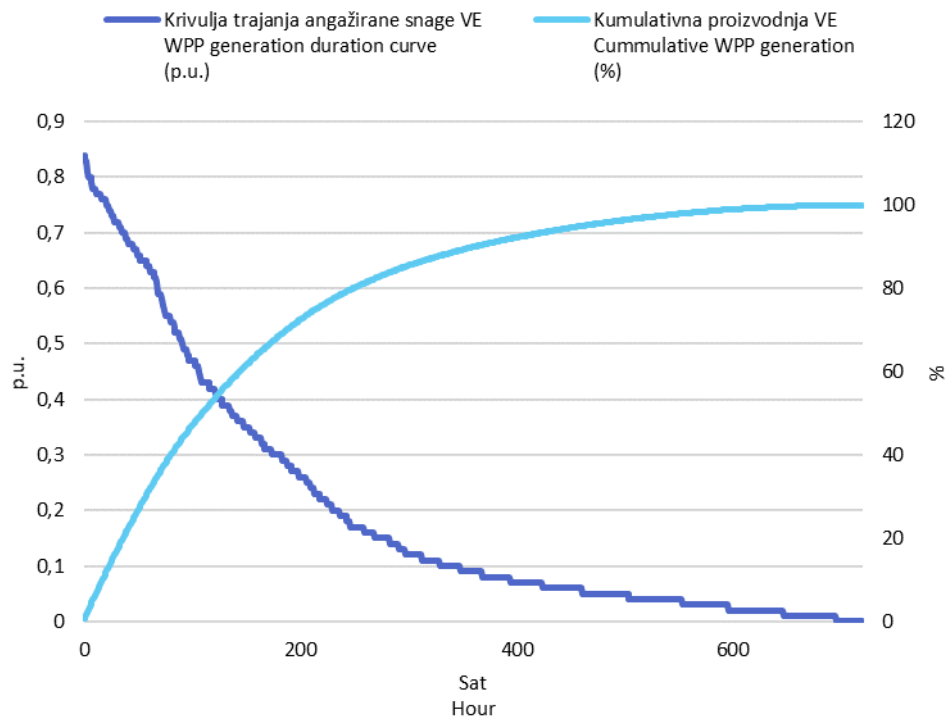
Slika 3 Krivulja trajanja angažirane snage svih VE i kumulativna proizvodnja VE u lipnju 2022. godine u jediničnim vrijednostima
