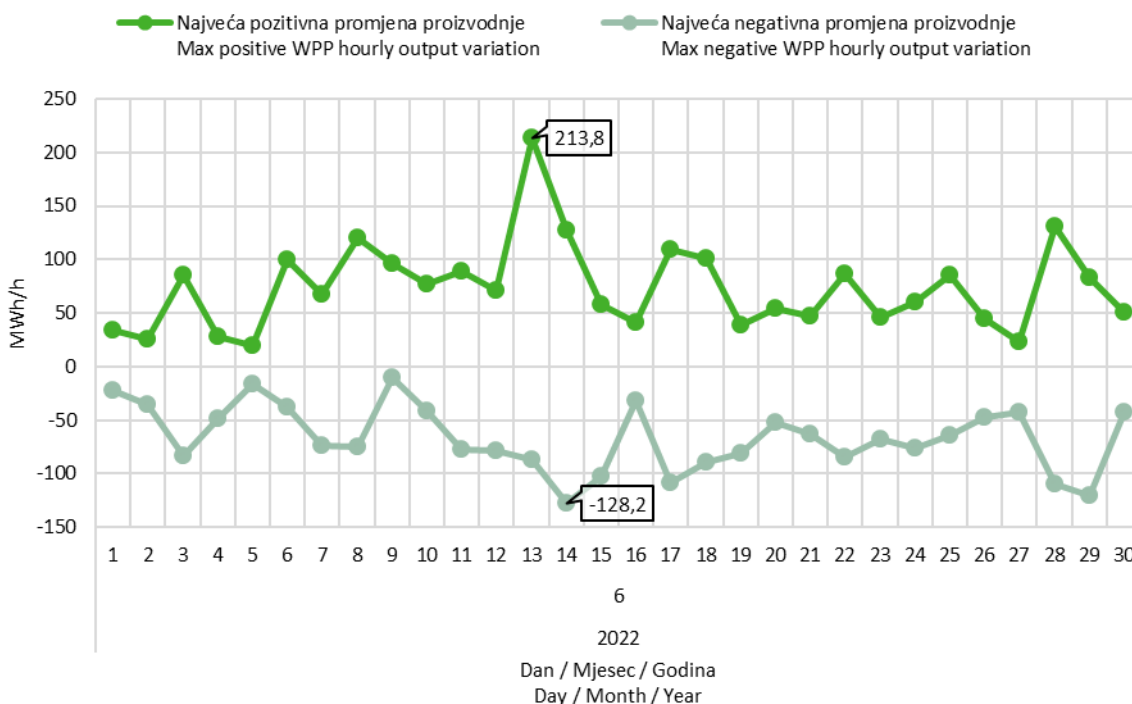
Slika 9 Maksimalna pozitivna i maksimalna negativna promjena satne proizvodnje VE u lipnju 2022. godine
